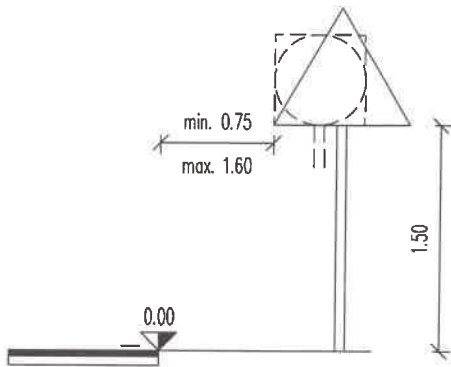
POSTAVITEV PZ OB CESTI IZVEN NASELJA
