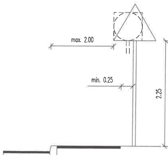
POSTAVITEV PZ OB CESTI V NASELJU S POVRŠINAMI ZA PEŠCE IN KOLESARJE
