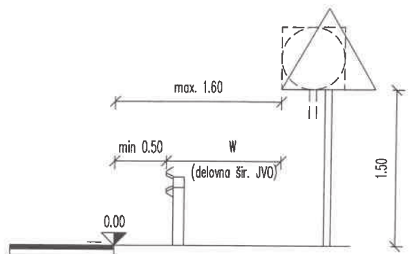
POSTAVITEV PZ PRI VARNOSTNI OGRAJI
