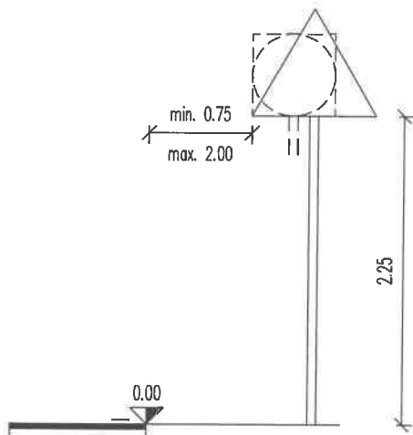
POSTAVITEV PZ OB CESTI V NASELJU
